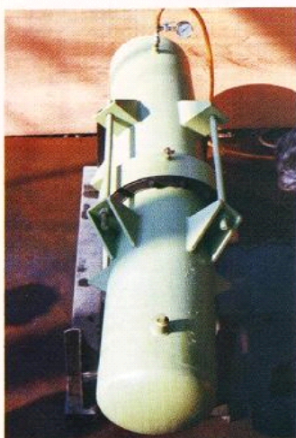
300A 撓角6° 漏水圧20kg/cm 2
