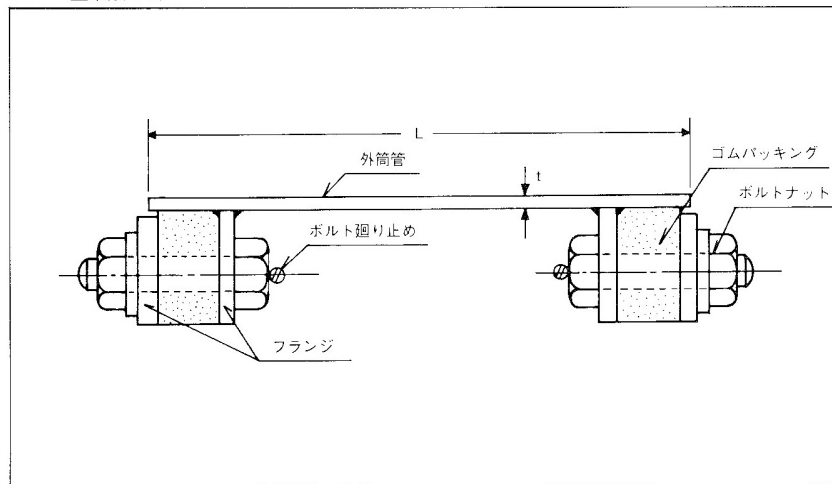
●Y-1型(鋼管用)
